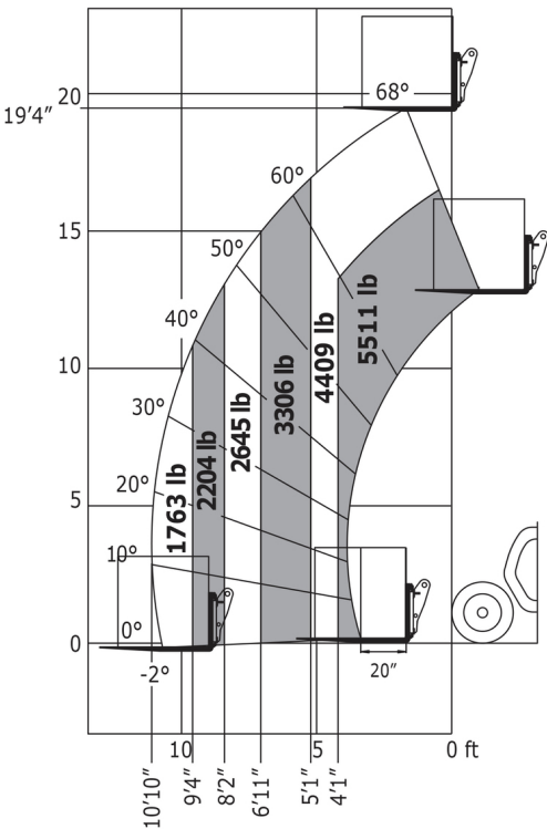
Macchina su pneumatici con forche Imperiale
