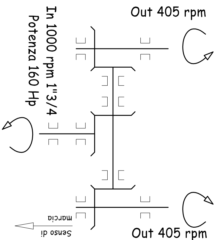
SCHEMA DI TRASMISSIONE MOTO
