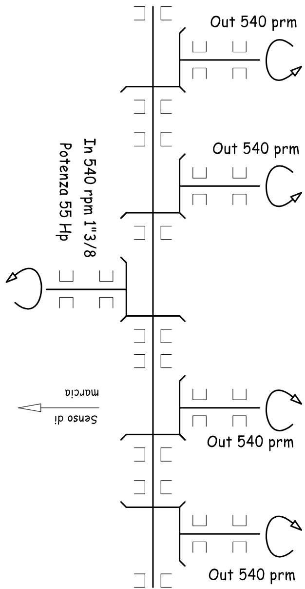
SCHEMA DI TRASMISSIONE MOTO
