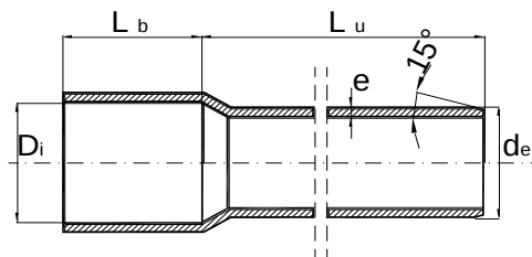
Tipo / Type G Bicchiere ad incollaggio Cement solvent socket Tulipe lisse à coller
