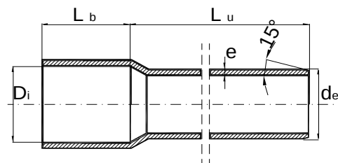
Tipo / Type B Bicchiere filettato M/F Threaded socket male/female tulipe fileté male/femelle
