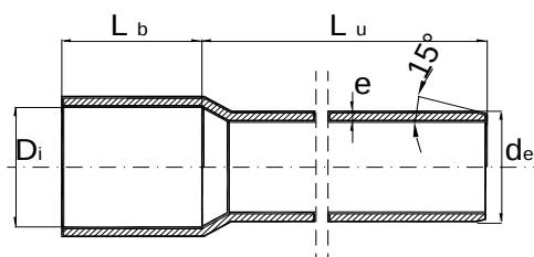
Tipo / Type B2 (2) Bicchiere filettabile, senza filetto Threadable socket, without threads tulipe à filer, non fileté
