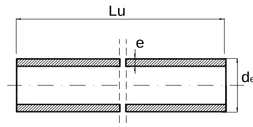
Tipo / Type T2 Estremità lisce Plain ends extrémité lisses
