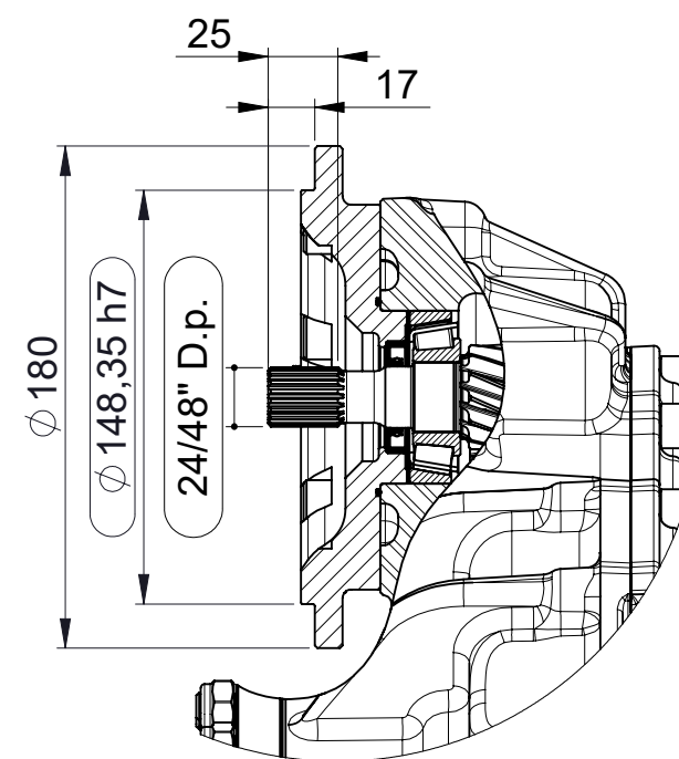
Flangia interfaccia trasmissione Transmission interface flange
