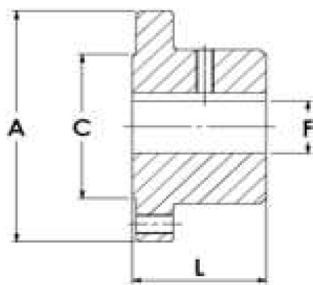
VERSIONE DIN DIN VERSION
