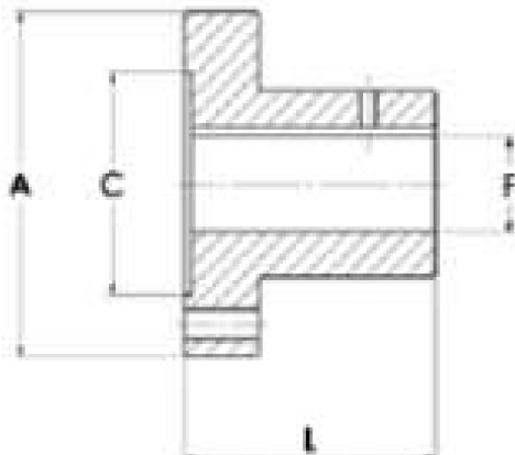
VERSIONE SAE SAE VERSION
