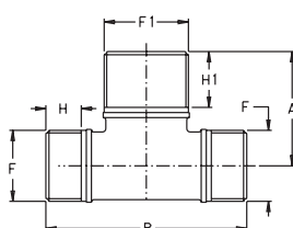
Raccordo a "T" filetti maschio per raccordi a battuta piana Male tee for flat seat fittings Raccord en "T" filetages mâle pour raccords avec siège plat
